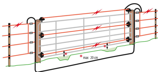
Bild 13 – Tor mit zusätzlicher Elektrifizierung als Schutz vor Untergraben bzw. Überklettern (Grafik: G. Herkert, Bild: F. Faß)
