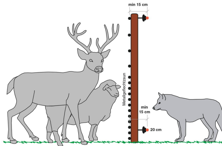
Bild 18 – Absicherung eines Stabzaunes mit 2 stromführenden Leitern (Grafik: G. Herkert)
